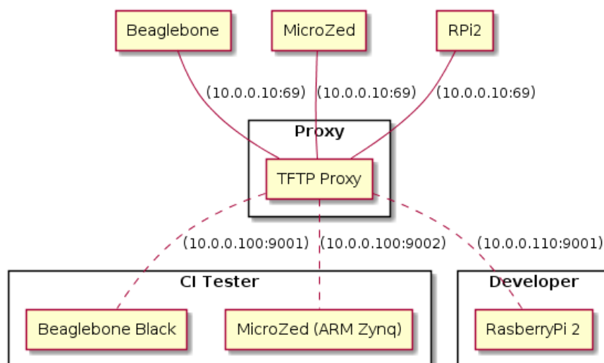
Fig. 13.1: RTEMS TFTP Proxy Test Lab
